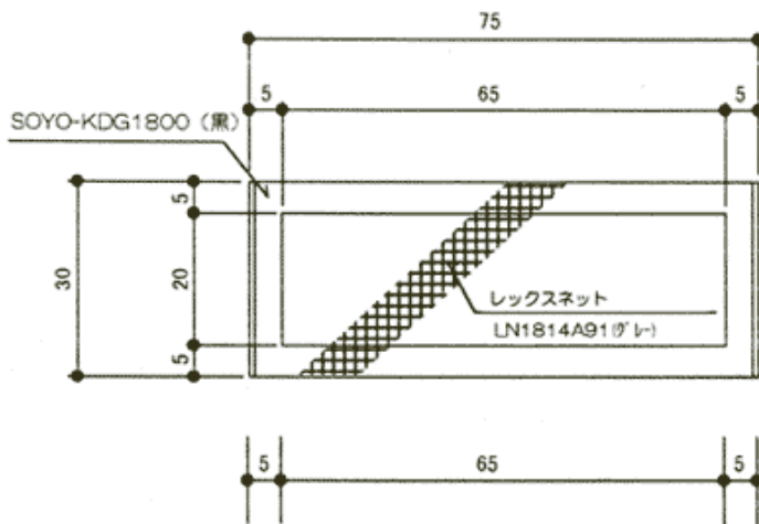
正面図 S1:1
